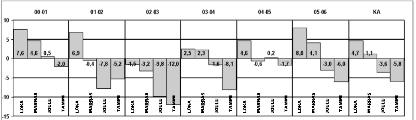
Yllä: Vanhakyläläisen Timo Karjakinin aamuisin 6 - 7 aikaan tehtyihin lämpötilahavaintoihin perustuva keskiarvokaavio.
